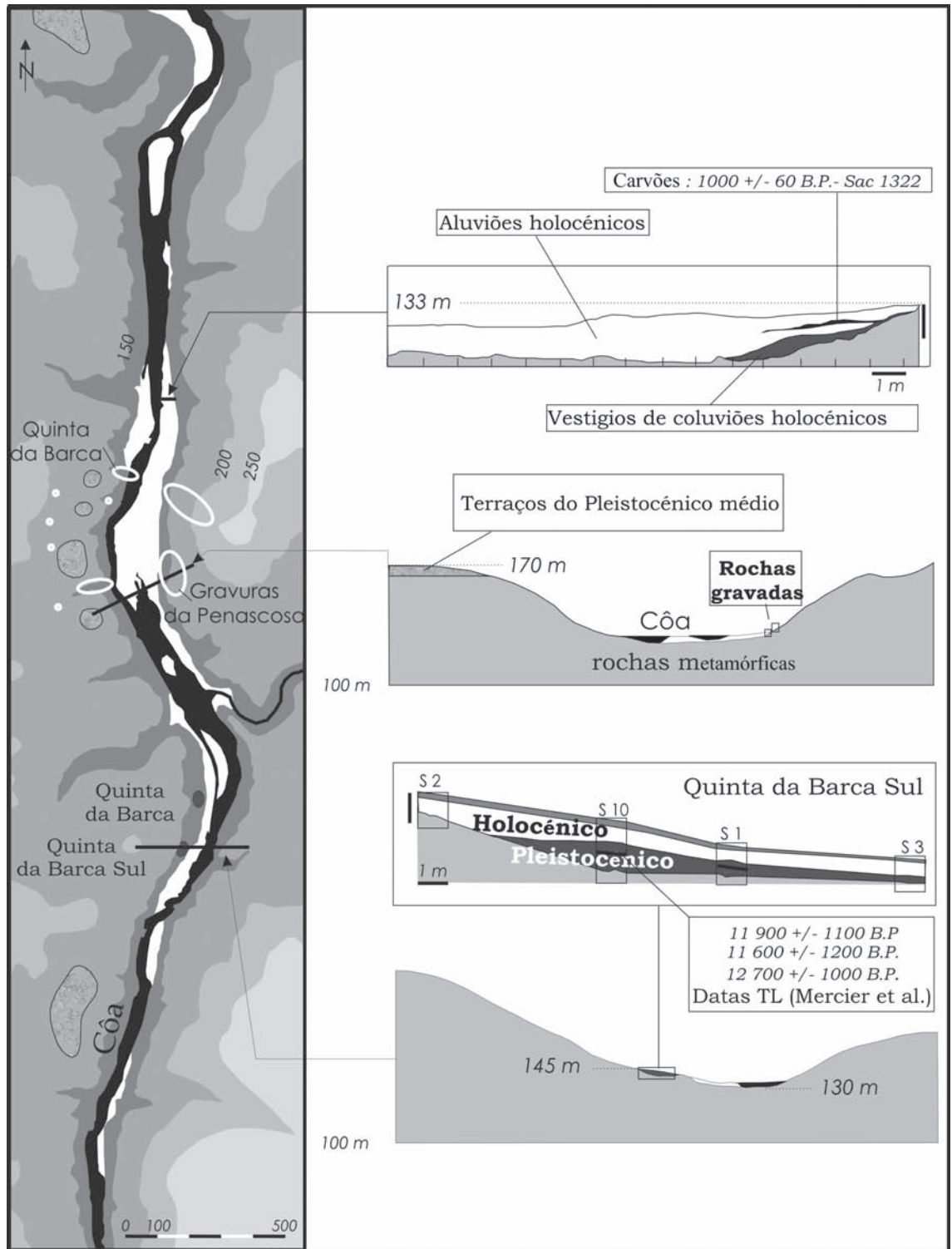
FIG. 4.1-2 – Posição e organização estratigráficas dos conjuntos sedimentares pleistocénicos e holocénicos no troço do Côa área da Quinta da Barca e da Penascosa.
