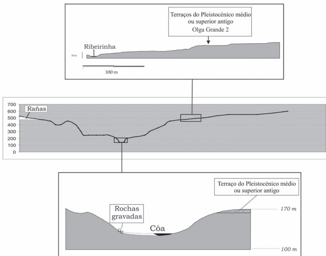
FIG. 4.1-1 – Perfis topográficos perpendiculares ao curso do Côa e do seu afluente, Ribeirinha. Observam-se as diferenças de cotas relativas das superfícies de aplanção em relação aos depósitos aluviais atribuíveis ao Pleistocénico médio ou superior antigo nos terrenos xistosos do fundo do Vale e na superfície de aplanção da Meseta.
