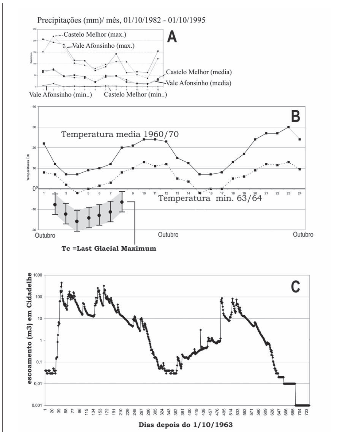
FIG. 2.4A - Precipitação média (mensal) entre 1982 e 1995 em Castelo Melhor e Vale Afonsinho, B: Temperatura média e mínima (mensal) e reconstituição das temperaturas médias dos meses mais frios durante o Último Máximo Glaciário, C: Escoamento depois de 1/10/1963 em Cidadelhe.
