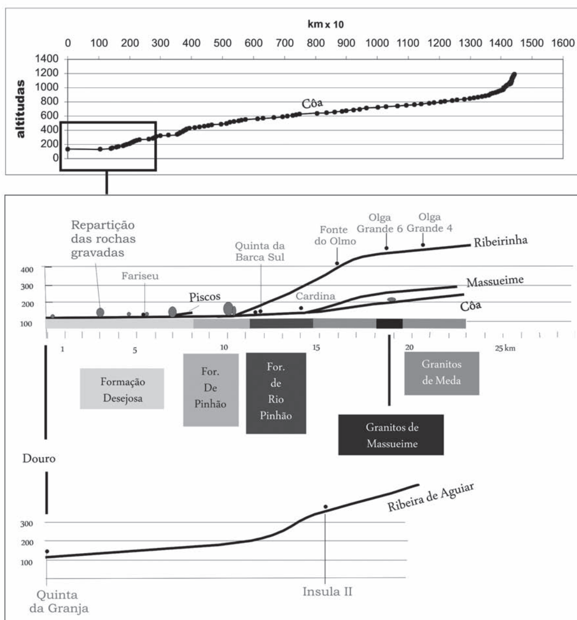
FIG. 2-2 - Perfil longitudinal do Rio Côa e dos seus afluentes nos seus últimos 25 km, com as formações geológicas percorridas.
